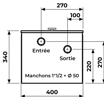
VUE CÔTÉ RACCORDEMENTS
